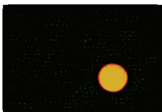
Merkury
