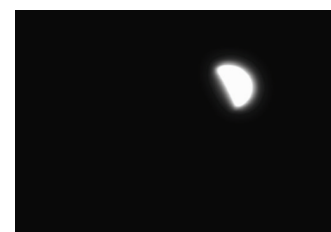
Venus
