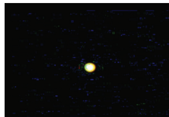
Uran
