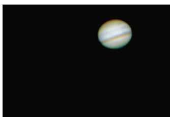
Jowisz
