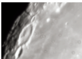
Księżyc
